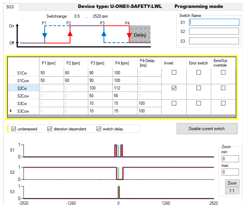
Abb. 4-7: Konfiguration UO-SGS-R
