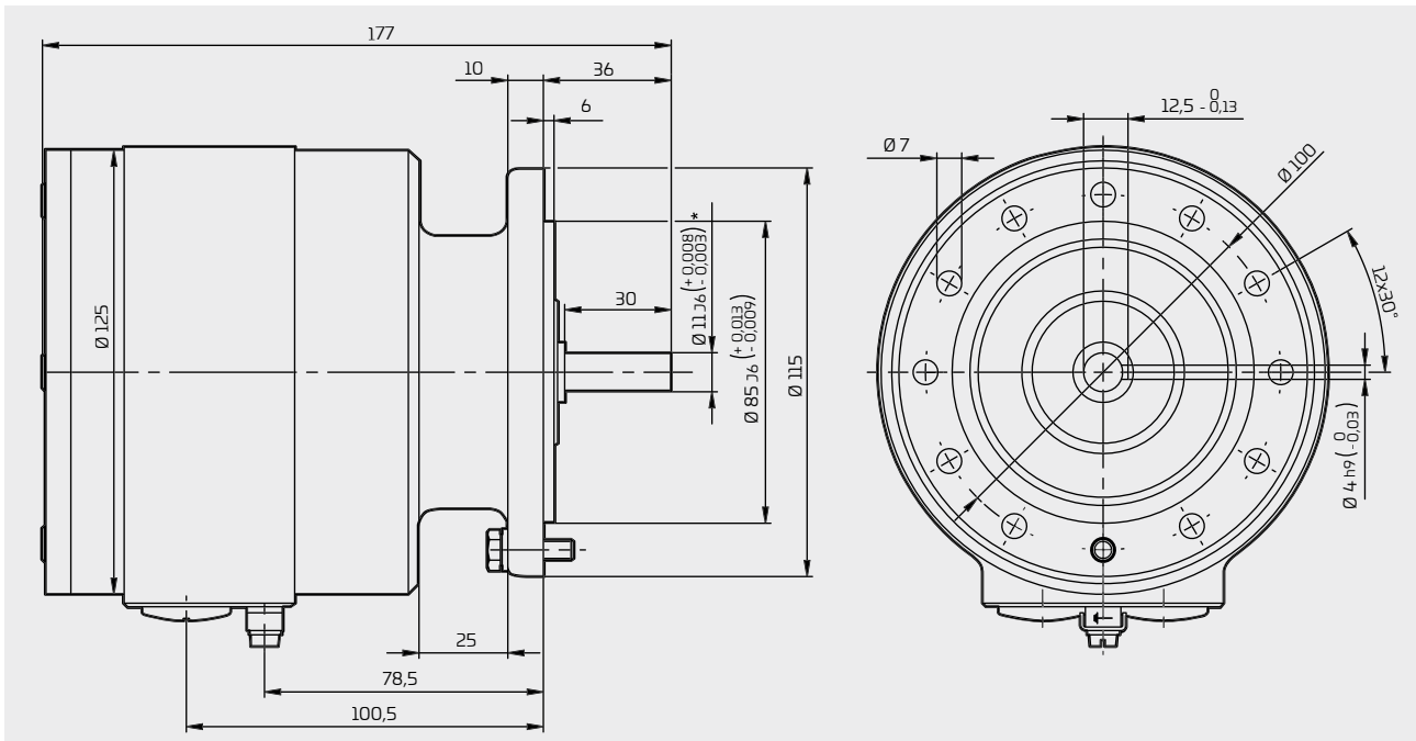
FG 40 Ex Bauform B5 Construction type B5
