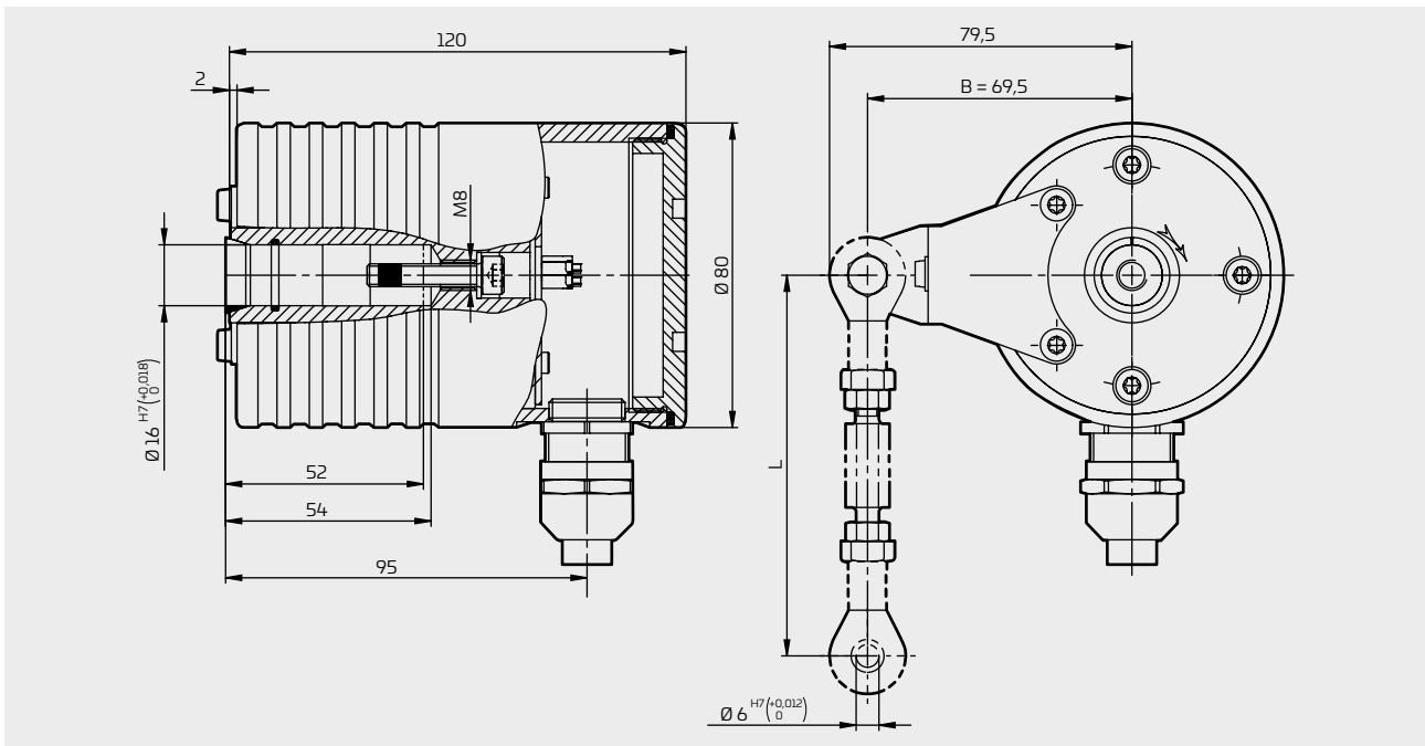
FGHJ INOX Hohlwellen-Bauform mit gestrichelter Drehmomentstütze Hollow shaft design with torque bracket indicated by dashed line
