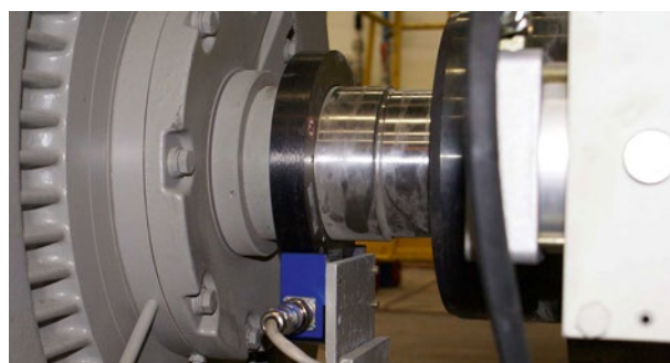
Дооснащение без демонтажа благодаря разъемному магнитному кольцу / Retrofit without removal of installation due to split pulse wheel
