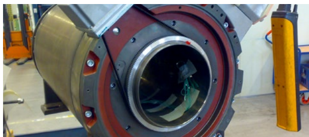
До: внешний датчик с зубчатым ремнем; проблемы с сигналом из-за вибрации зубного ремня / Before: external encoder with tooth belt; signal problems through tooth belt vibration
