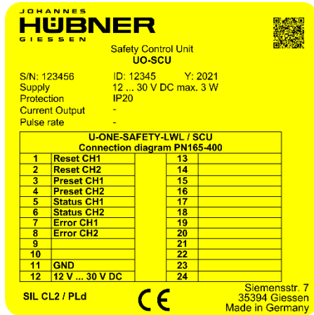
Abb. 4-1: Typenschild (Beispiel)
