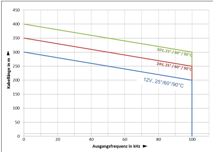
Abbildung 4: : Maximal zulässige Kabellänge bei TTL-Schnittstelle
