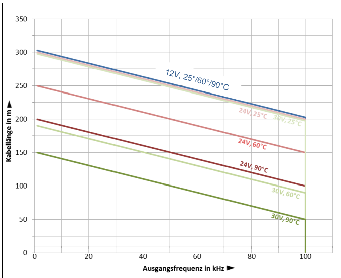
Abbildung 5: : Maximal zulässige Kabellänge bei HTL-Schnittstelle
