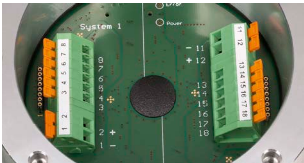
Klemmkasten Option AKK (zweiter Inkrementalausgang) Terminal box option AKK (second incremental output)
